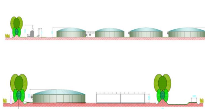
Figura 3. Sezioni Impianto di progetto
