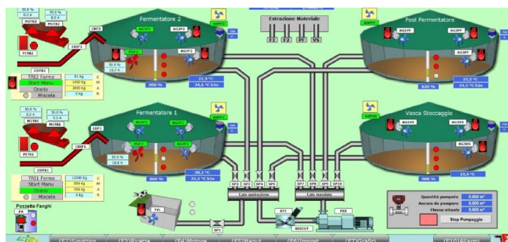
Figura 2. Schema funzionamento impianto
