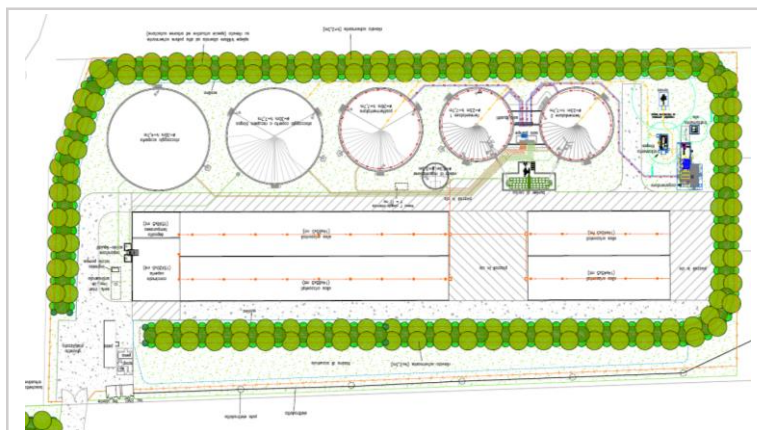
Figura 1. Progetto impianto a biogas
