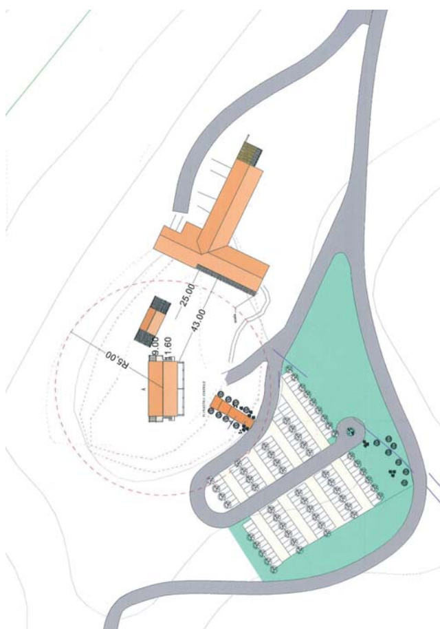
Planimetria di progetto del nuovo edificio rurale
