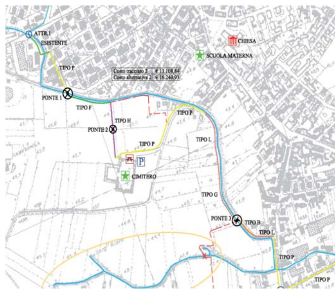
Stralcio di planimetria di progetto
