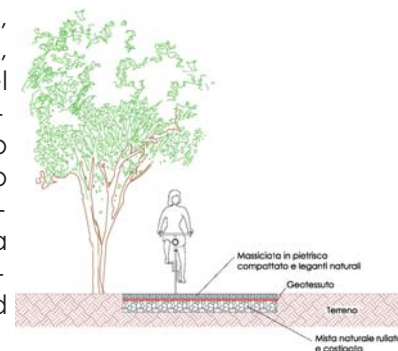
Sezione pista ciclabile
